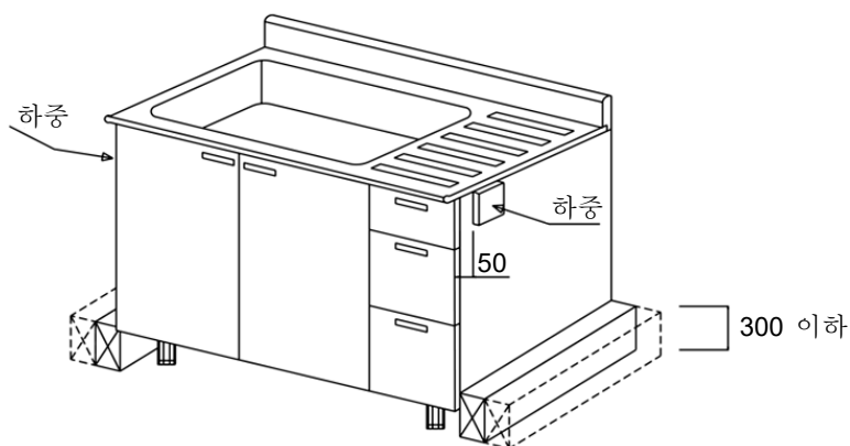
그림 7 — 강성 시험
