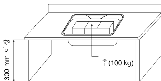
그림 9 — 언더상판의 싱크볼 조립강도 시험
