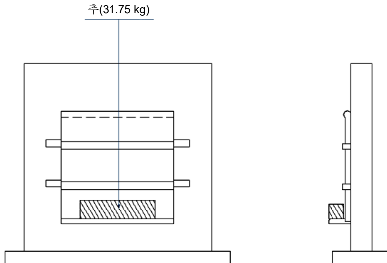
그림 13 — 포스트포밍(P/F) 테이블 위판 뒤턱 견고성 시험
