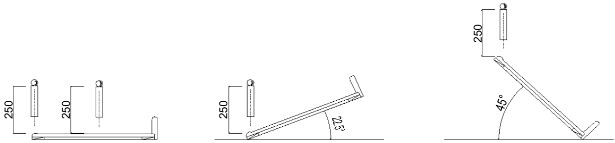
그림 12 — 포스트포밍(P/F) 테이블 위판 충격강도 시험
